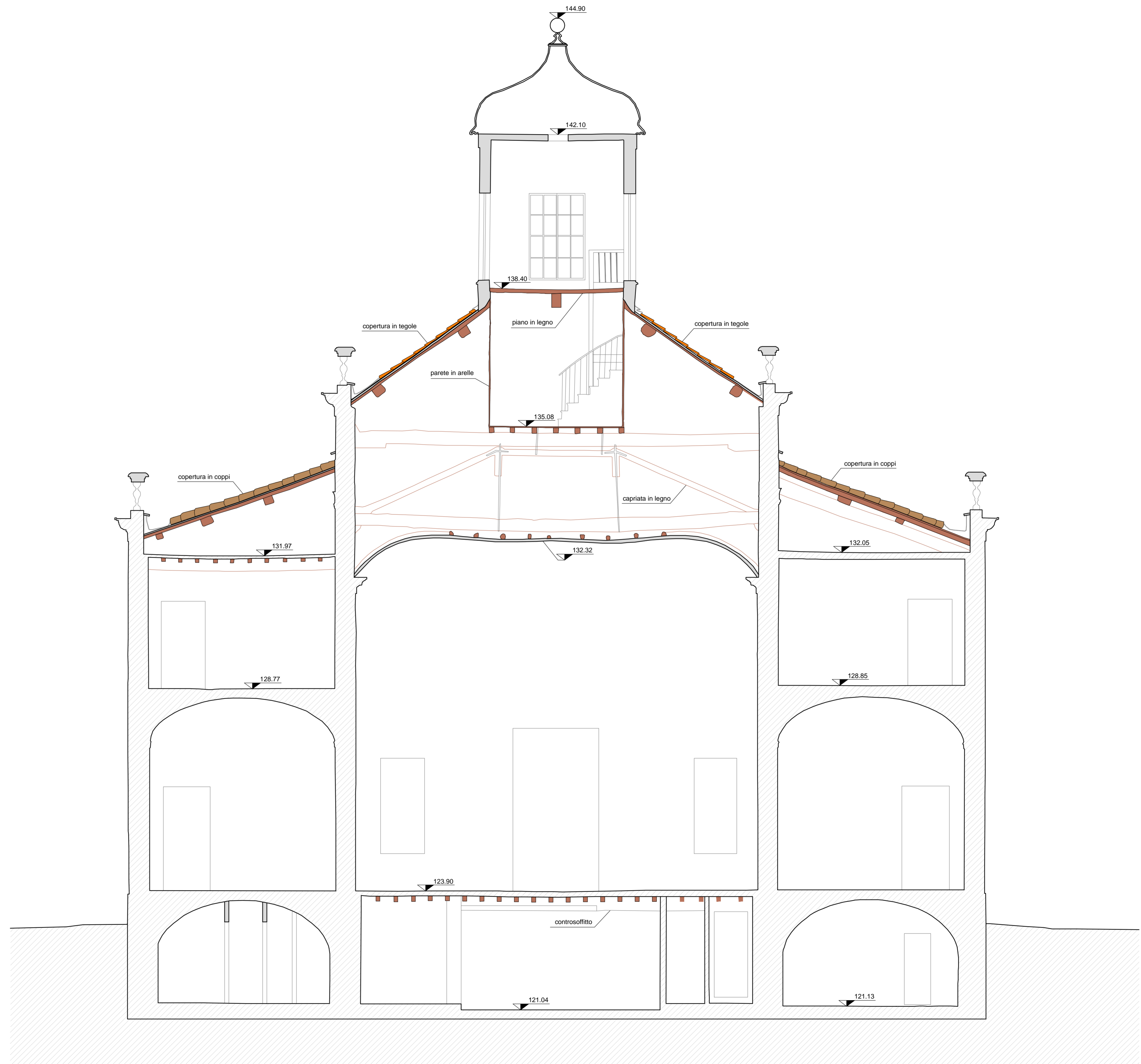
Seziona a-a
